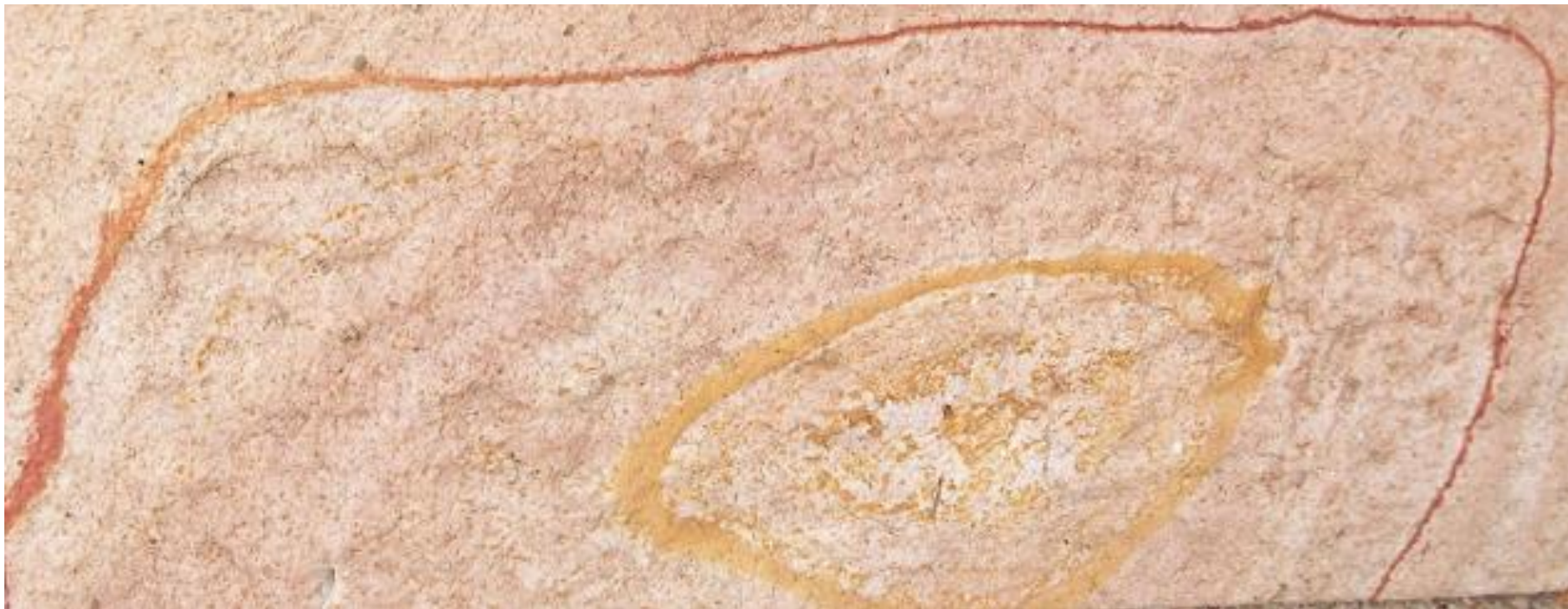
Линейные знаки и ареалы
